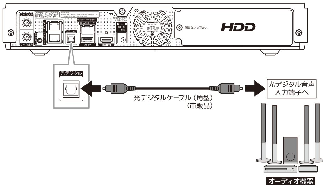
本機背面
