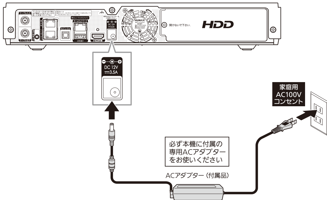
本機背面
